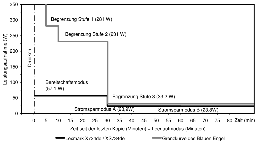
Leistungsaufnahme und Aktivierungszeiten der Lexmark X734de / XS734de während der seit dem letzten Druckauftrag verstrichenen Zeit nach dem letzten Druckauftrag
