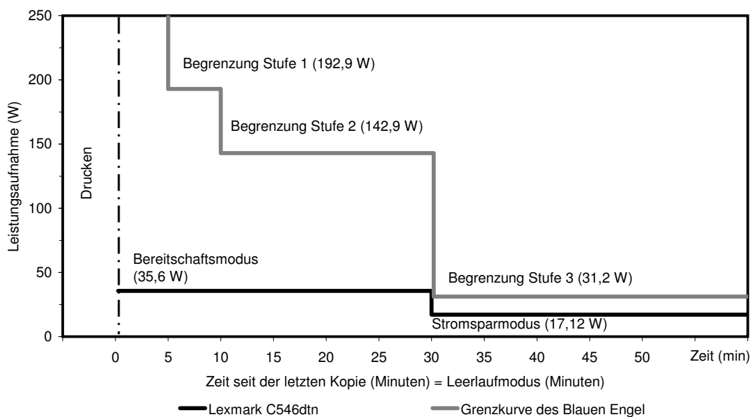
Leistungsaufnahme und Aktivierungszeiten des Lexmark C546dtn während der seit dem letzten Druckauftrag verstrichenen Zeit nach dem letzten Druckauftrag
