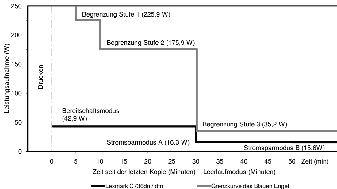
Leistungsaufnahme und Aktivierungszeiten der Lexmark C736dn / dtn während der seit dem letzten Druckauftrag verstrichenen Zeit nach dem letzten Druckauftrag
