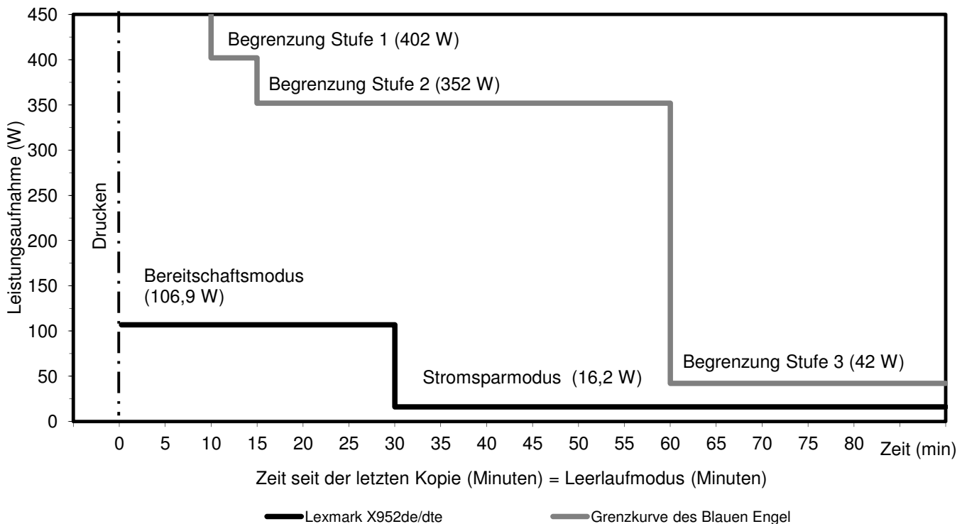
Leistungsaufnahme und Aktivierungszeiten der Lexmark X952de/dte während der seit dem letzten Druckauftrag verstrichenen Zeit nach dem letzten Druckauftrag
