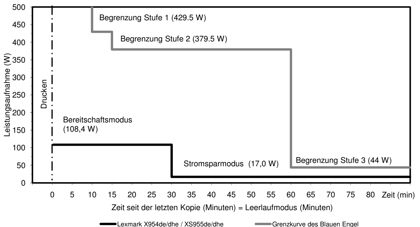
Leistungsaufnahme und Aktivierungszeiten der Lexmark X954de/dhe / XS955de/dhe während der seit dem letzten Druckauftrag verstrichenen Zeit nach dem letzten Druckauftrag
