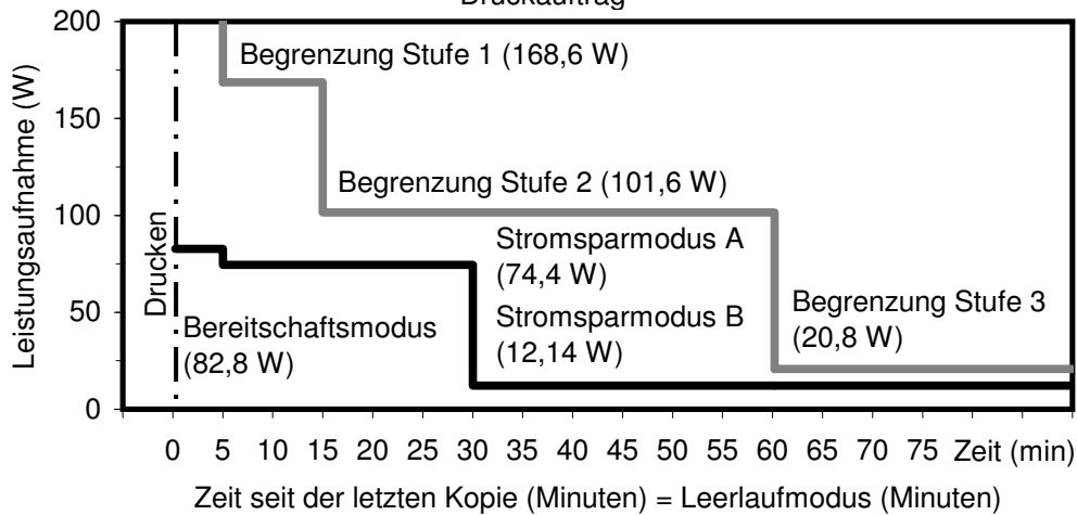
Leistungsaufnahme und Aktivierungszeiten der Lexmark T652dn / dtn während der seit dem letzten Druckauftrag verstrichenen Zeit nach dem letzten Druckauftrag
