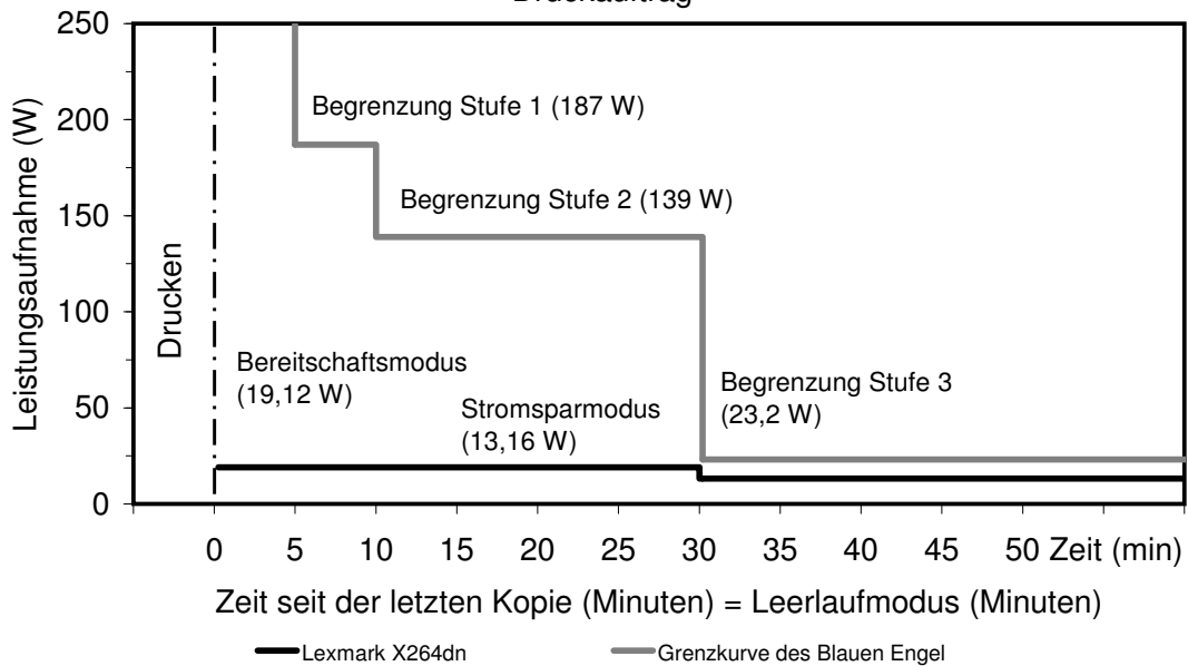
Leistungsaufnahme und Aktivierungszeiten des Lexmark X264dn während der seit dem letzten Druckauftrag verstrichenen Zeit nach dem letzten Druckauftrag
