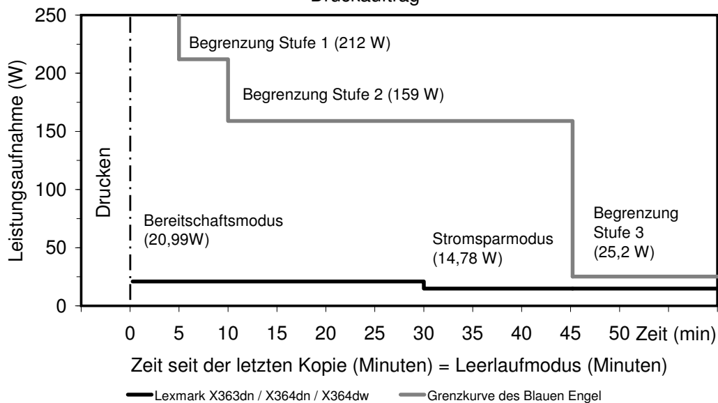
Leistungsaufnahme und Aktivierungszeiten der Lexmark X363dn / X364dn /X364dw während der seit dem letzten Druckauftrag verstrichenen Zeit nach dem letzten Druckauftrag
