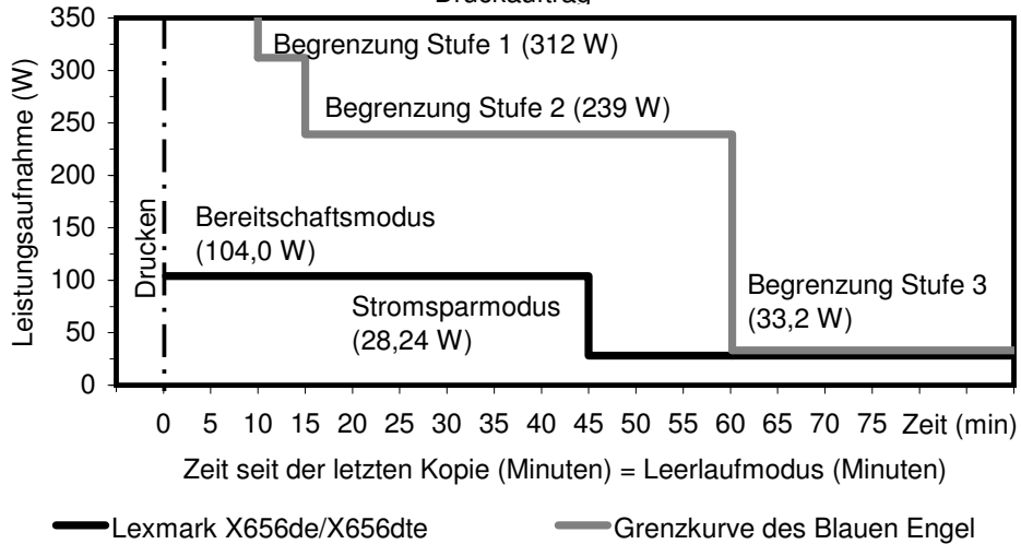
Leistungsaufnahme und Aktivierungszeiten der Lexmark X656de / X656dte während der seit dem letzten Druckauftrag verstrichenen Zeit nach dem letzten Druckauftrag
