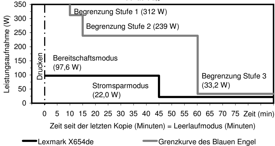
Leistungsaufnahme und Aktivierungszeiten des Lexmark X654de während der seit dem letzten Druckauftrag verstrichenen Zeit nach dem letzten Druckauftrag
