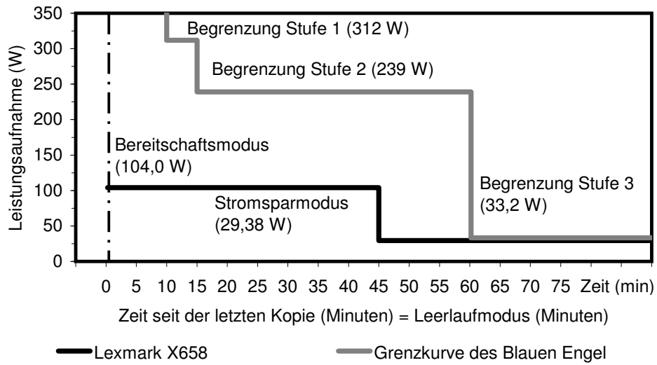
Leistungsaufnahme und Aktivierungszeiten der Lexmark X658 während der seit dem letzten Druckauftrag verstrichenen Zeit nach dem letzten Druckauftrag
