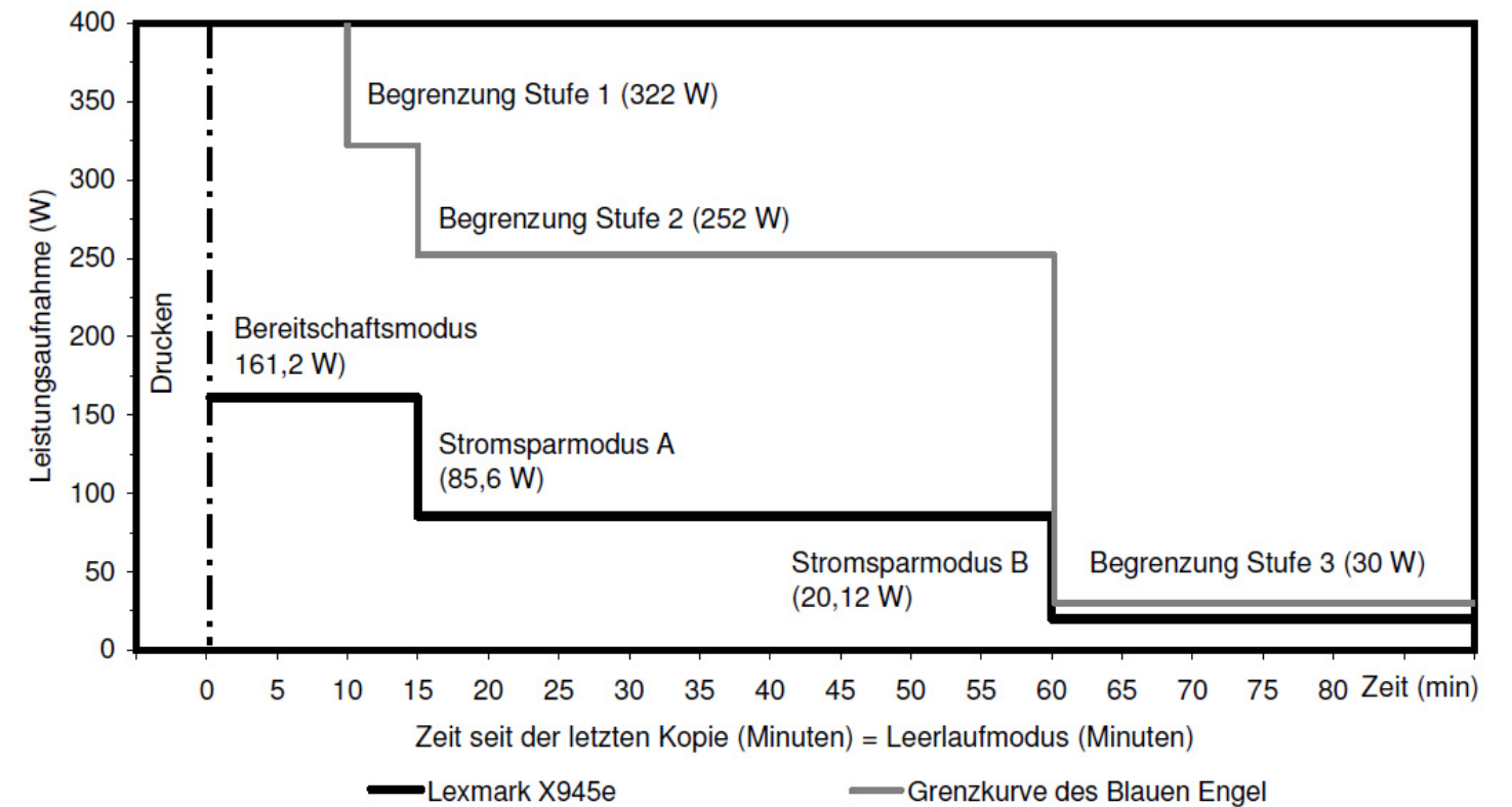
Leistungsaufnahme und Aktivierungszeiten des Lexmark X945e während der seit dem letzten Druckauftrag verstrichenen Zeit nach dem letzten Druckauftrag
