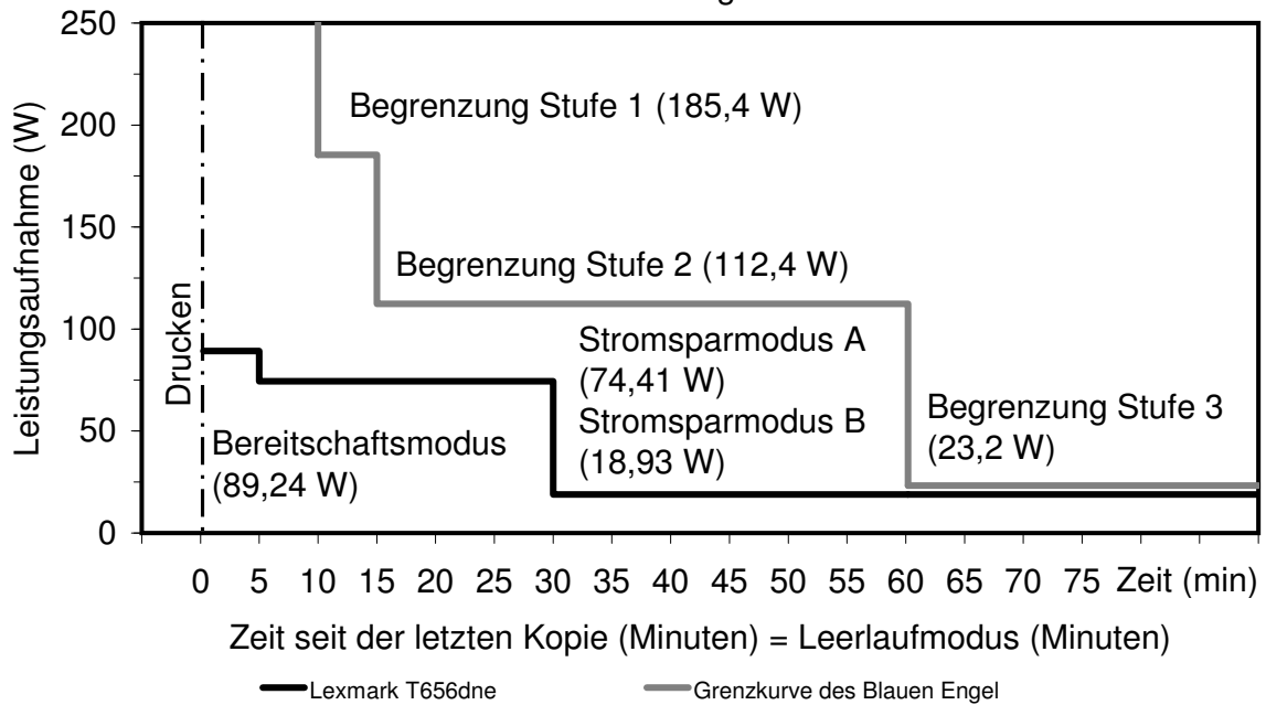
Leistungsaufnahme und Aktivierungszeiten des Lexmark T656dne während der seit dem letzten Druckauftrag verstrichenen Zeit nach dem letzten Druckauftrag
