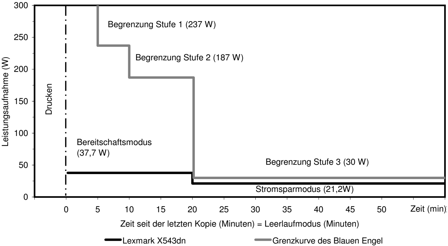
Leistungsaufnahme und Aktivierungszeiten des Lexmark X543dn während der seit dem letzten Druckauftrag verstrichenen Zeit nach dem letzten Druckauftrag
